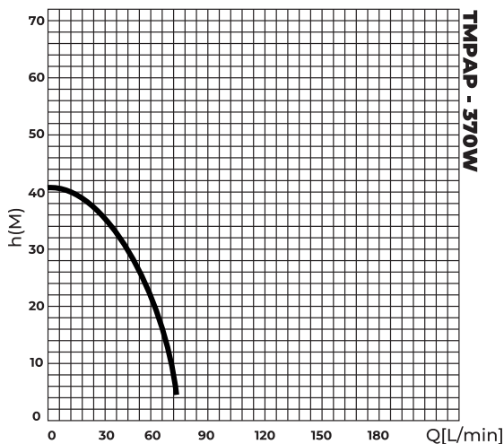
Grafico pressão x vazão
